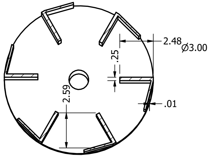
SECTION A-A SCALE 6 : 1
